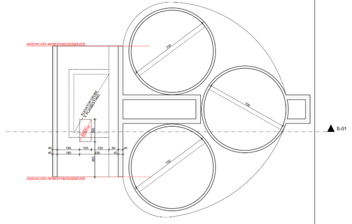
ERDGESCHOSS - DARSTELLUNG II. PLANBESTAND - M 1:100
